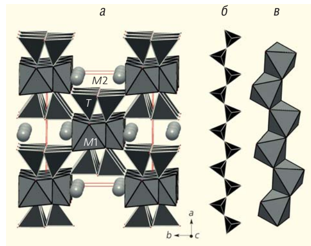
Рис.2. Структура минералов группы пироксена: каркас ( a ), (Si,O)-цепочка ( b ) и O -лента ( в ).
