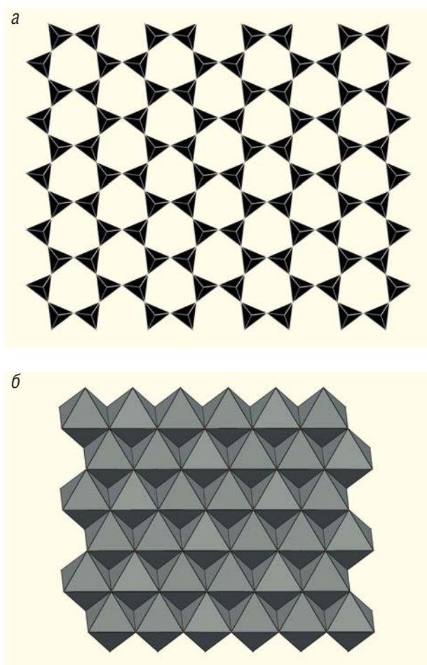
Рис.5. Тетраэдрический (Si,O)-слой (а) и октаэдрический O-слой (б) в структуре минералов группы слюд.
