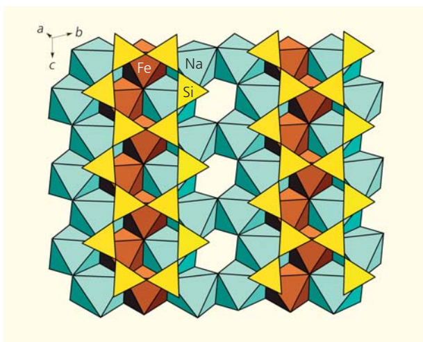
Рис.11. Структура ершовита: O -слой из октаэдров Fe и Na и амфиболовые (Si,O)-ленты.
